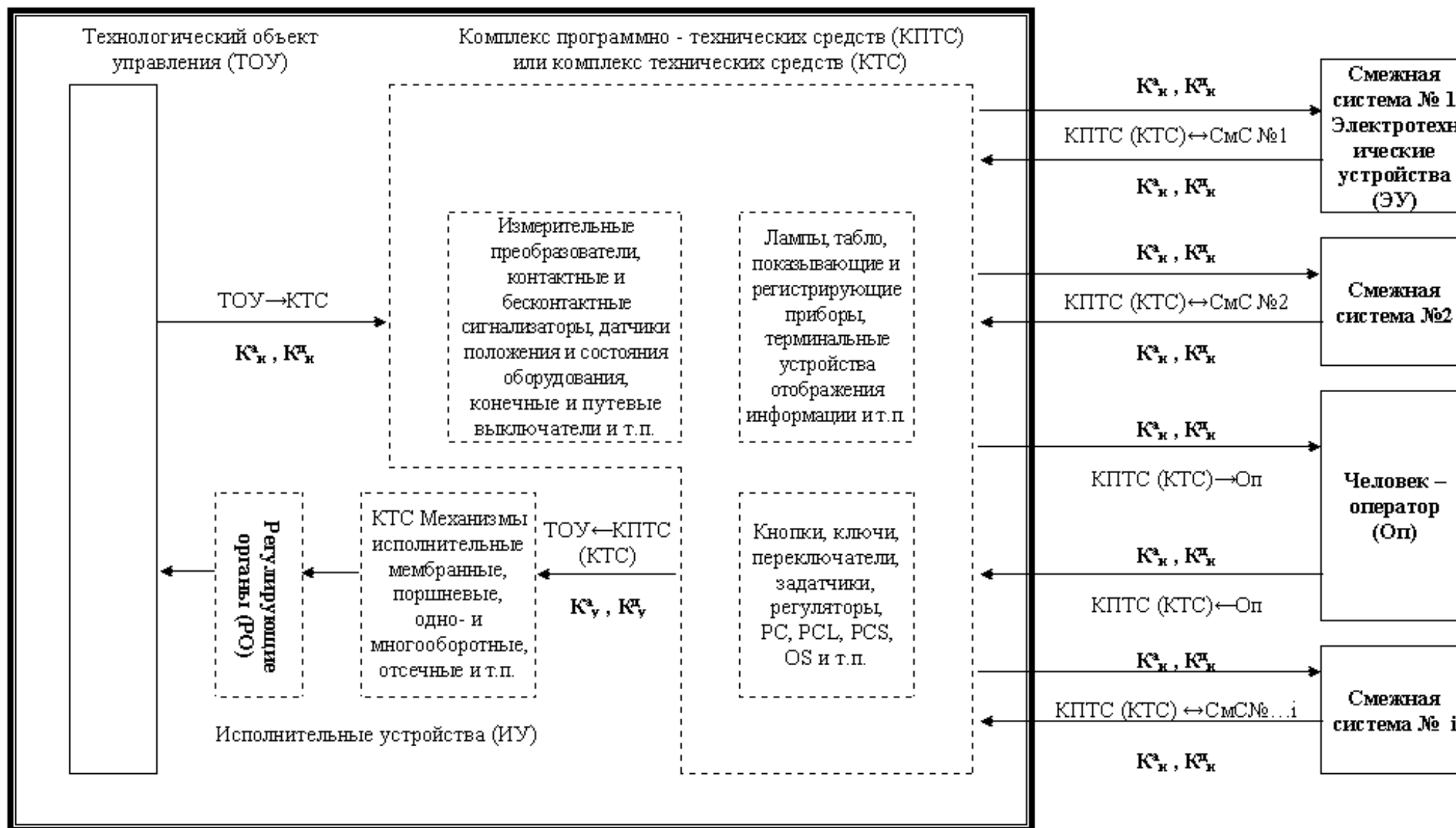
Схема автоматизированного технологического комплекса (АТК)
